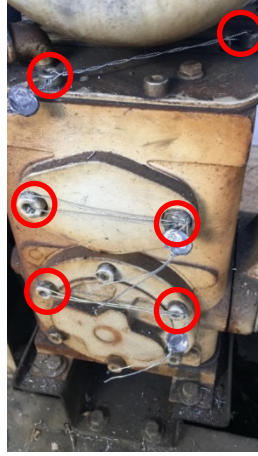
Şekil 12 Tip 2 Emişli Pompa Damgası
