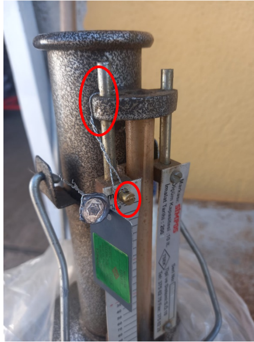
Şekil 2 Hacim Ölçek Kabı Gösterge Damgalaması
