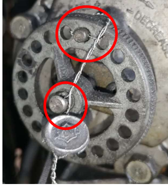
Şekil 6 Brodimetre Ayar Çarkı Damgası
